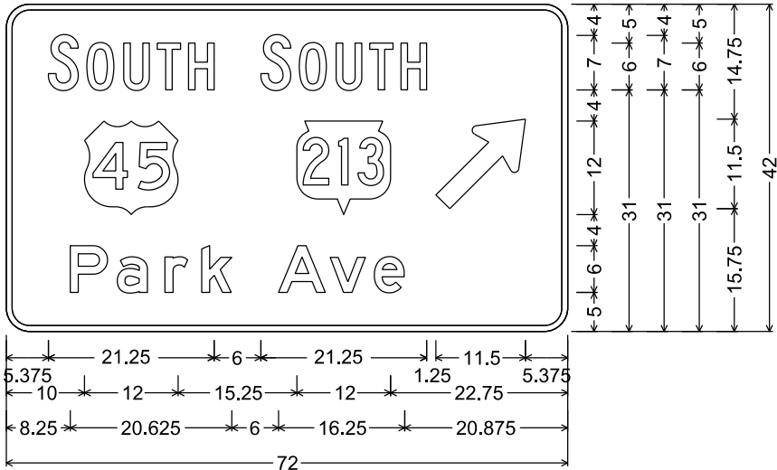
D1-1F; 3.000" Radius, 0.750" Border
