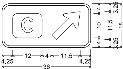
D1-1E; 3.000" Radius, 0.750" Border
