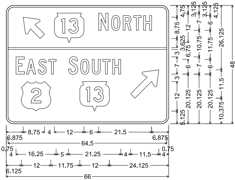
D1-1G; 3.000" Radius, 0.750" Border
