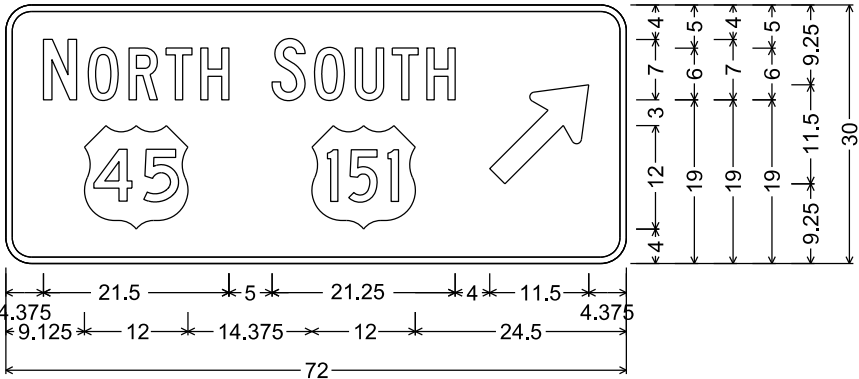
D1-1F; 3.000" Radius, 0.750" Border
