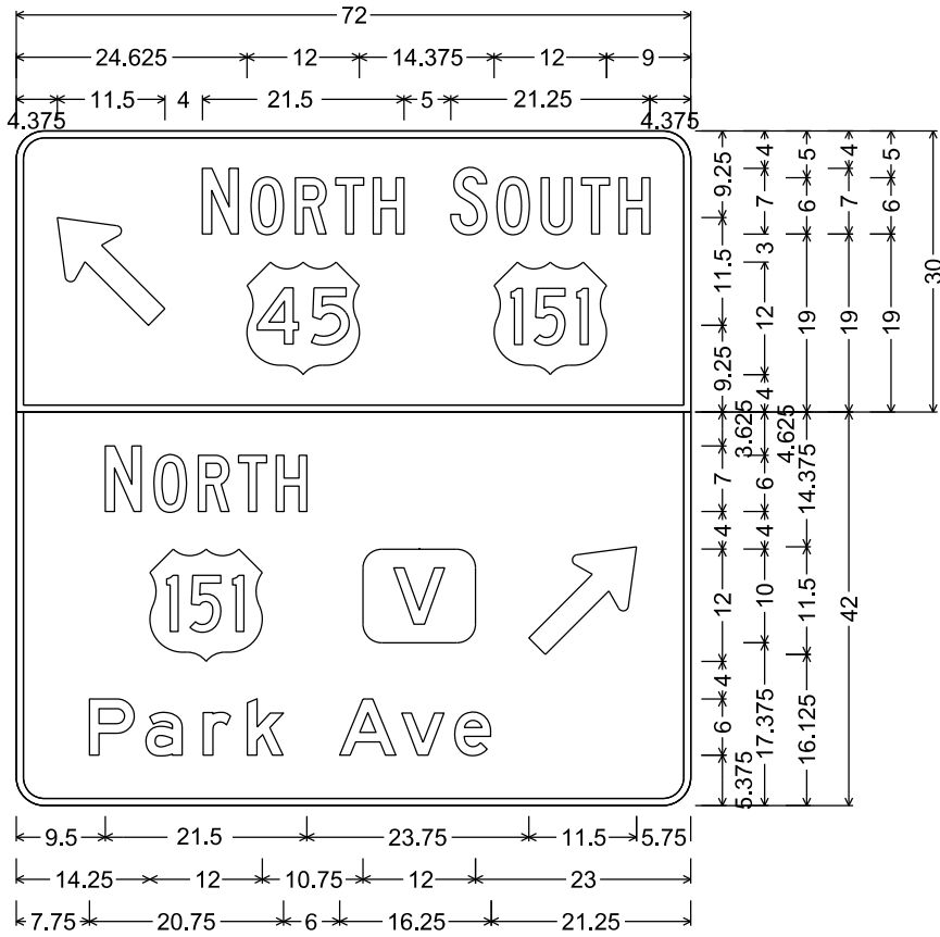
D1-1G; 3.000" Radius, 0.750" Border
