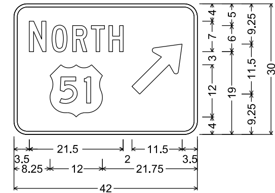
D1-1E; 3.000" Radius, 0.750" Border
