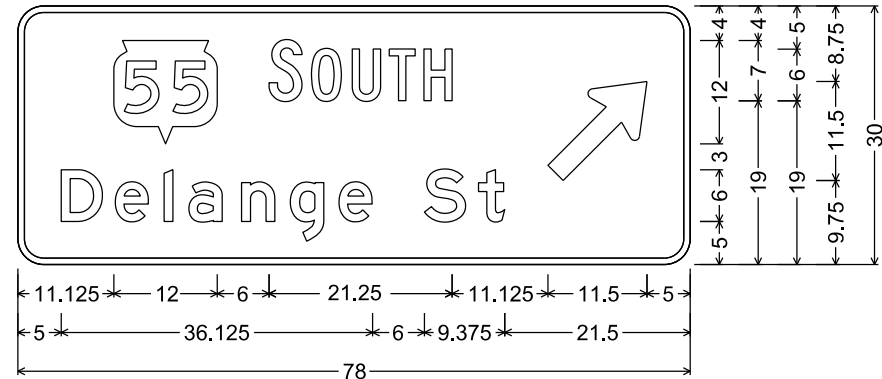
D1-1F; 3.000" Radius, 0.750" Border
