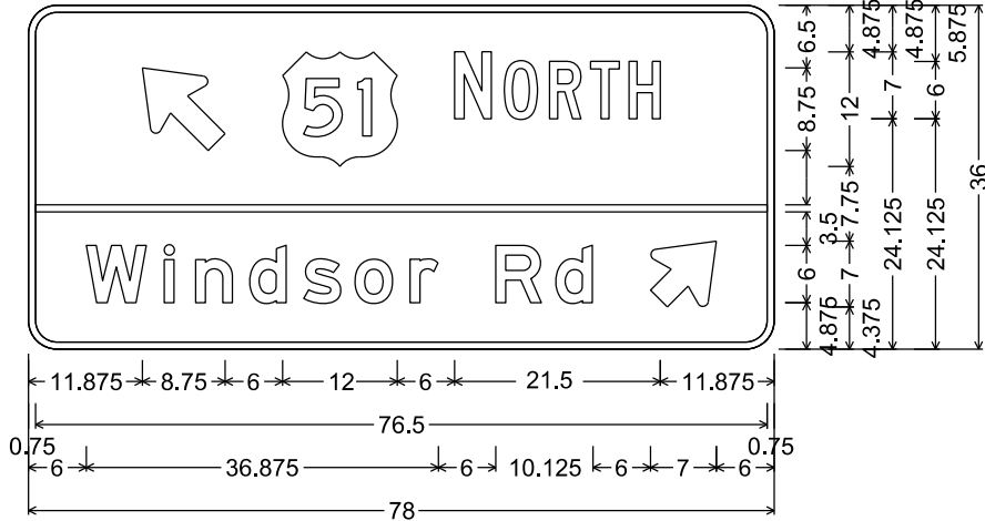
D1-1F; 3.000" Radius, 0.750" Border
