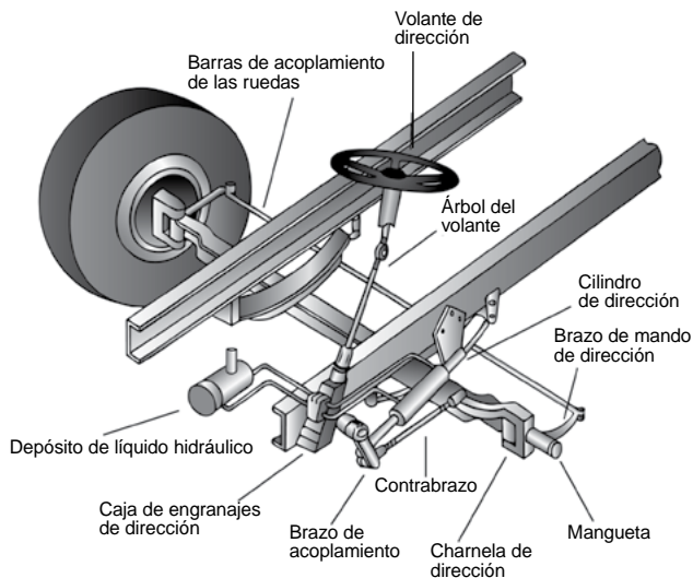
Figura 2-1: Piezas Claves del Sistema de Dirección
